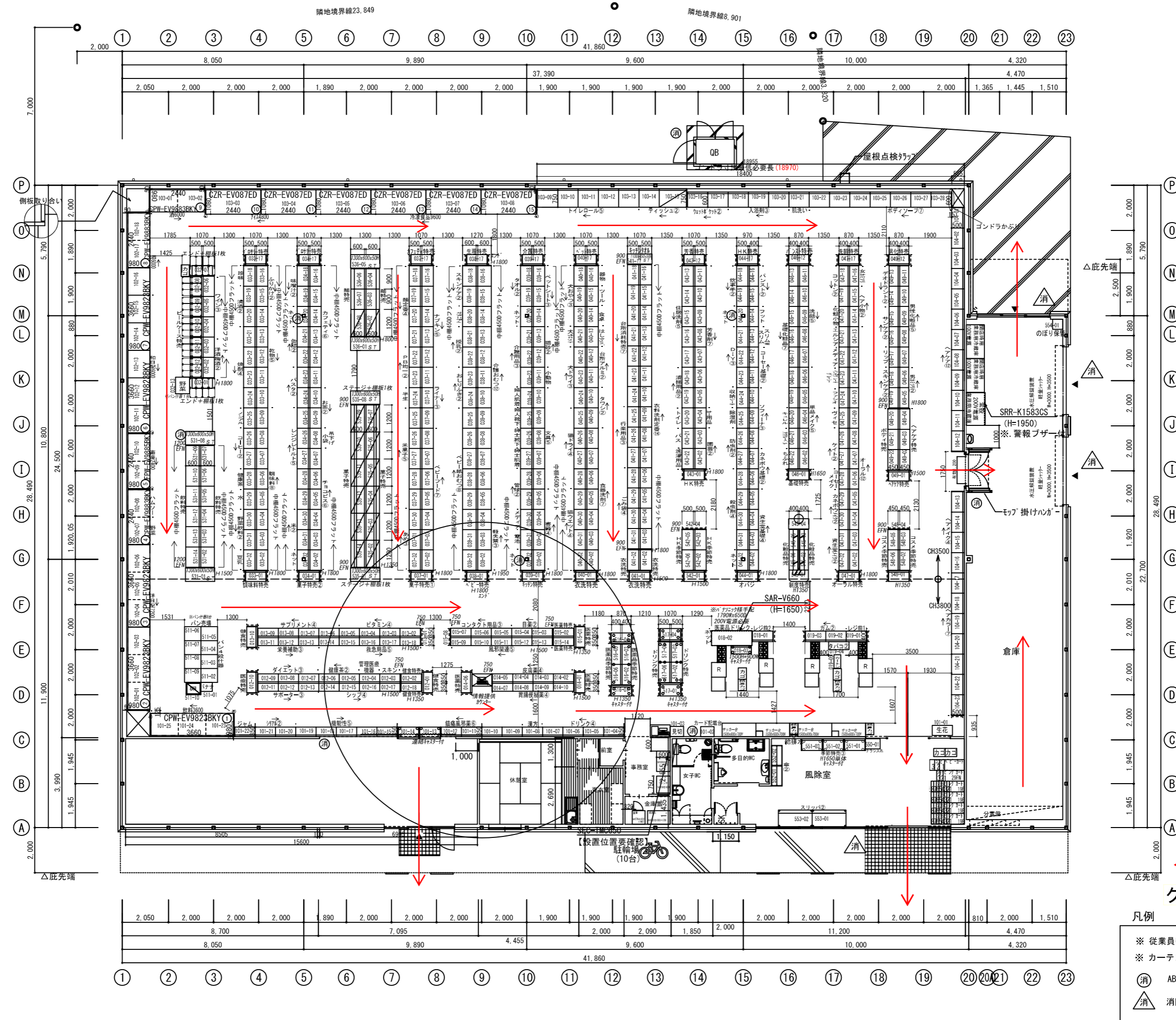
平面図 S=1:100
